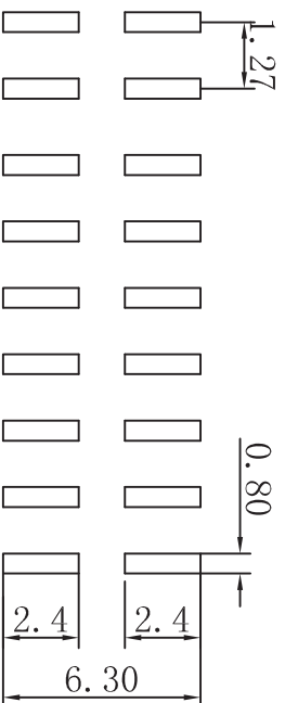
P.C.B LAYOUT
