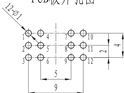
PCB板开孔图
